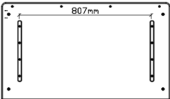
top(俯视图)
