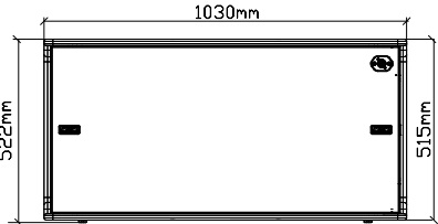
front(前视图)
